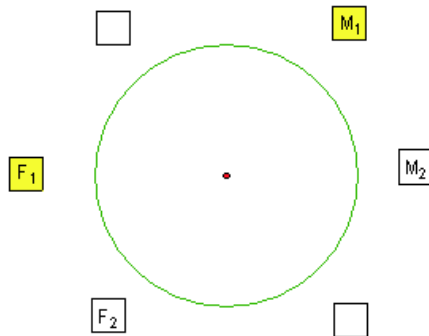
Abb. 3: Eine Möglichkeit für M_2
