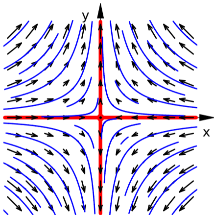
Linearisierung
