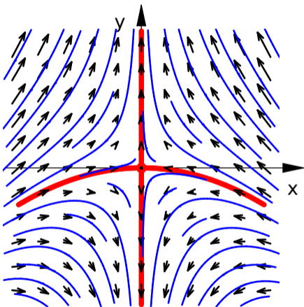
Nichtlineares System
