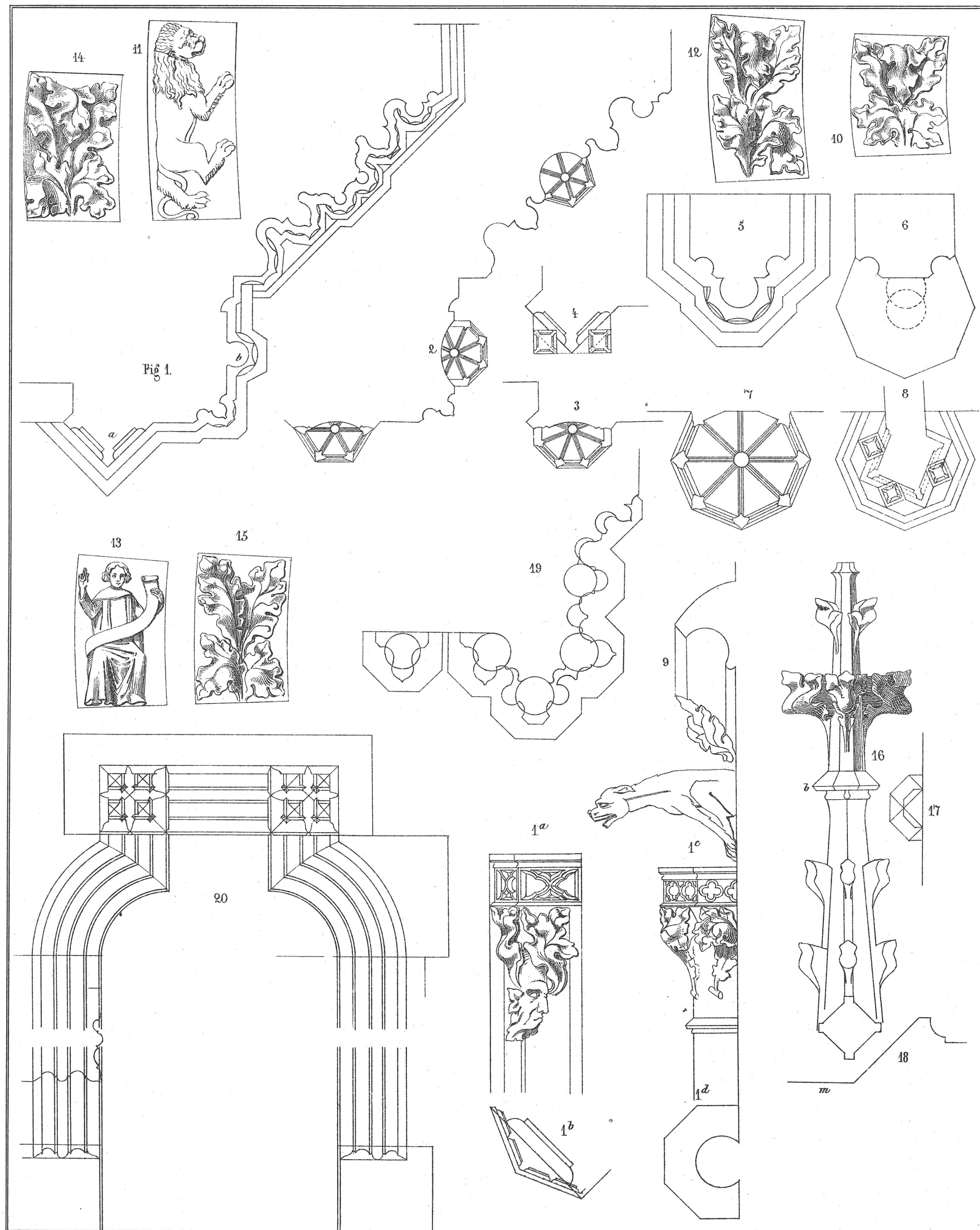
1—18. Einzelheiten zum Portal aus Homburg, siehe Tafel 17. — 19. Grundriß zu Tafel 16. — 20. Thür im Kreuzgang zu Haina.
