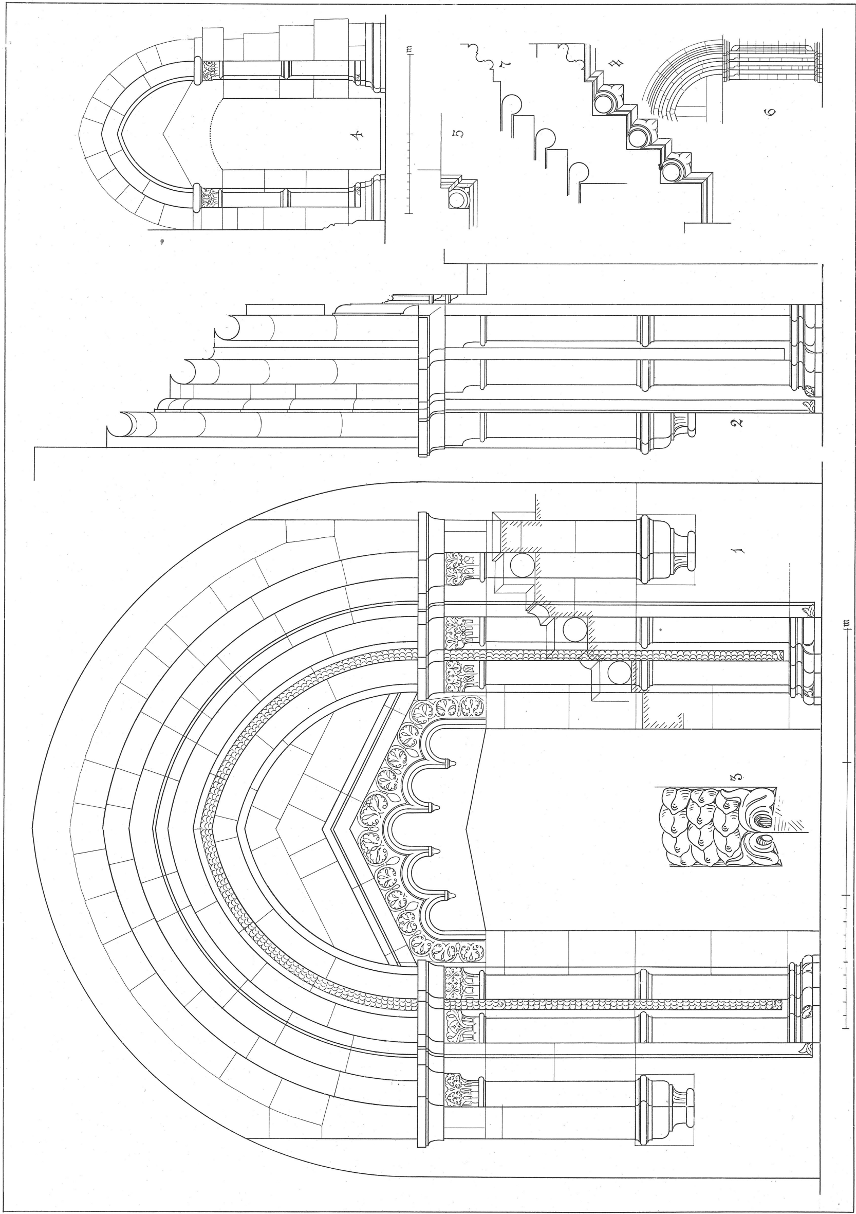
1—3. Portal aus Wieprechtshausen. — 4—5. Pforte aus Wieprechtshausen. — 6—8. Portal vom südl. Querschiff des Domes in Minden.
