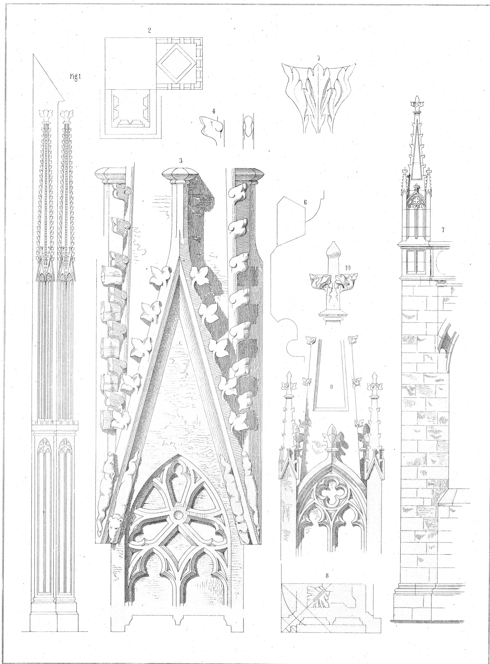
1—6. Strebe Pfeiler vom Grabdenkmal des Ulrich von Lichtenberg in Strassburg. — 7—10. Strebe Pfeiler von den Chorkapellen in Freiburg.
